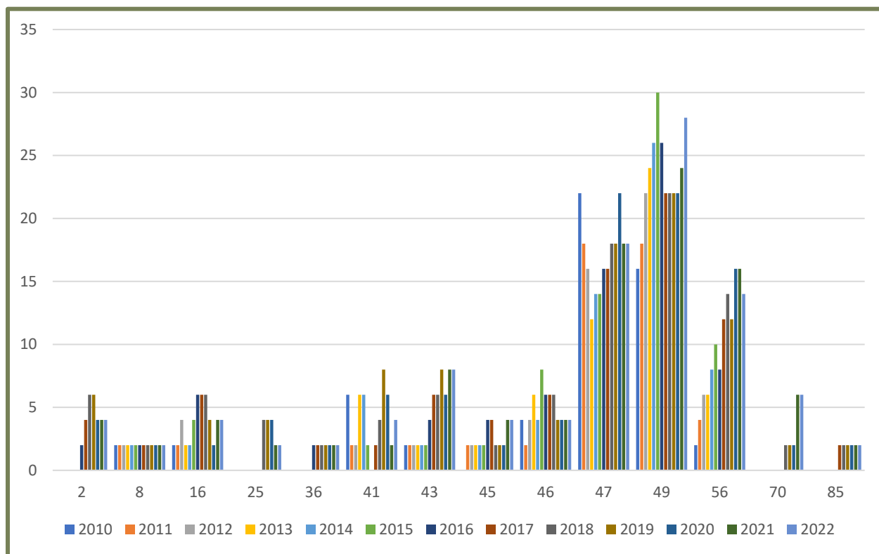
Figură 47 Dinamica numărului întreprinderilor active pe sectoare, în UAT Bărbătești, între anii 2010-2022
