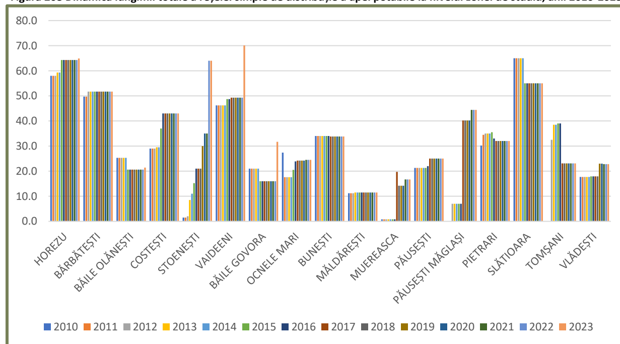
Figură 208 Dinamica lungimii totale a rețelei simple de distribuție a apei potabile la nivelul zonei de studiu, anii 2010-2023
