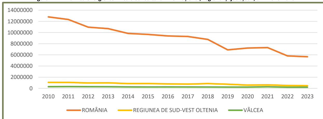
Figură 212 Dinamica energiei termice distribuite la nivel național, regional și județean, anii 2010-2023
