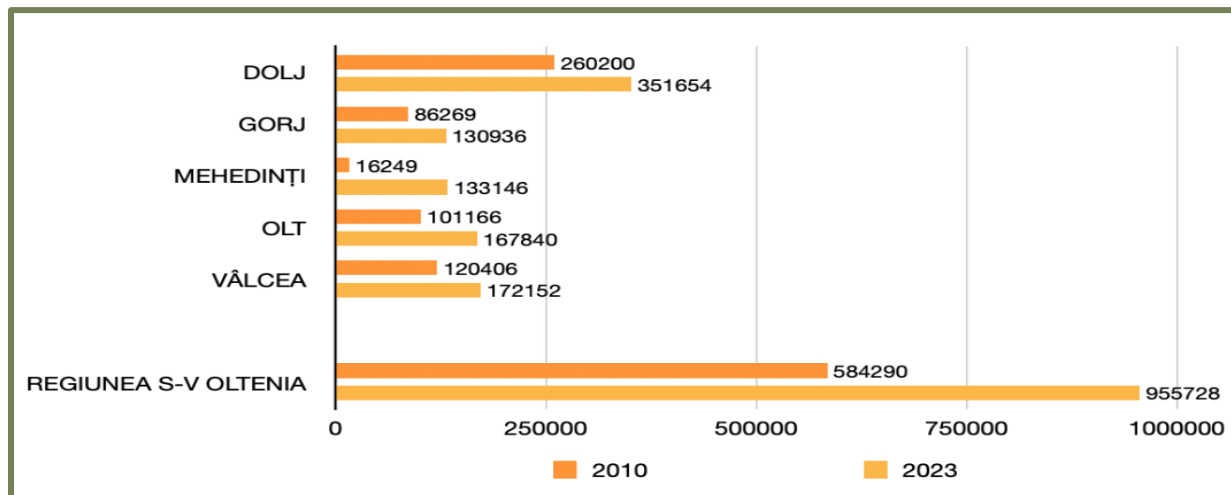
Figură 208 Populația conectată la sistemele de canalizare și epurare a apelor uzate (număr de persoane), la nivel județean și regional, în perioada 2010–2023
