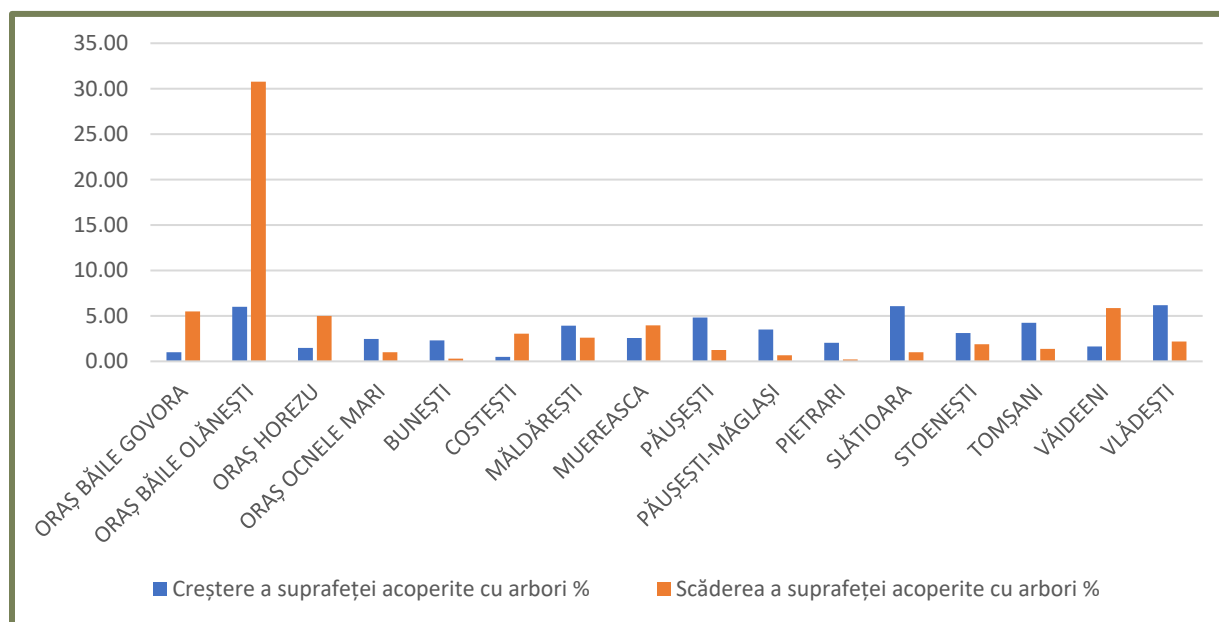
Figură 192 Creșterea suprafeței acoperite cu arbori (2000-2020) și pierderea suprafeței acoperite cu arbori (2001-2024)
