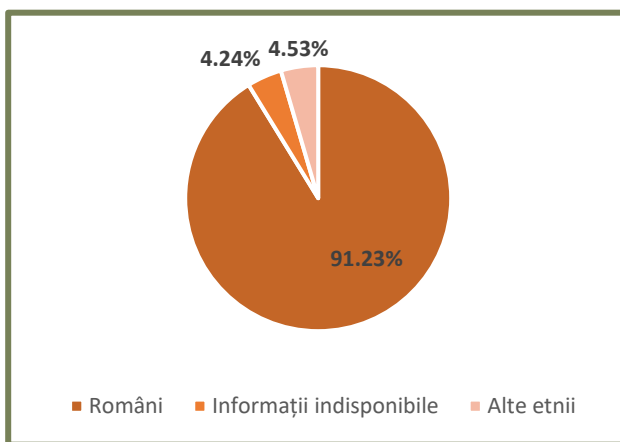
Figură 21 Populația la nivelul UAT-urilor din zona de studiu pe etnii, în anul 2024
